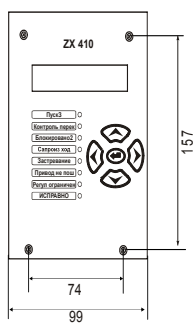
ВИД СПЕРЕДИ
