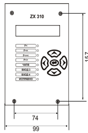
ВИД СПЕРЕДИ
