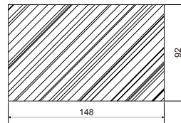
ВЫРЕЗАЕМОЕ ОТВЕРСТИЕ В ДВЕРИ РЕЛЕЙНОГО ШКАФА
