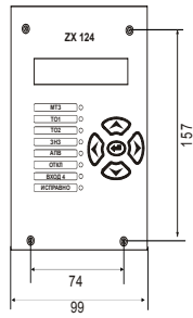
ВИД СПЕРЕДИ
