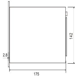
ВИД СБОКУ
