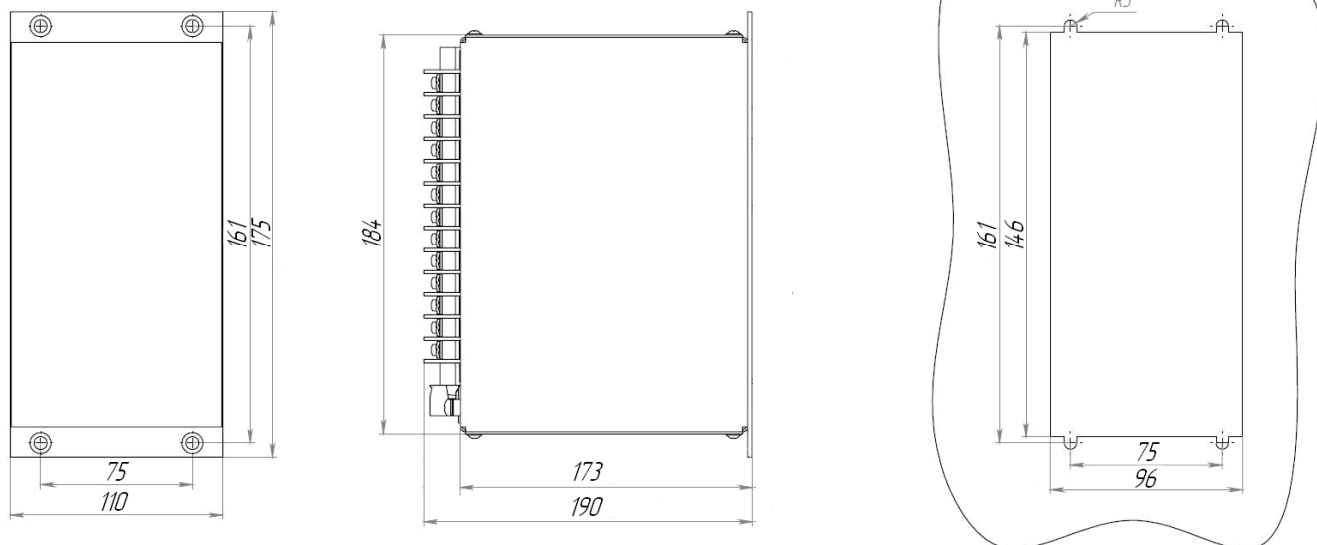
Габаритные и установочные размеры LX 120 РЕДУТ.
