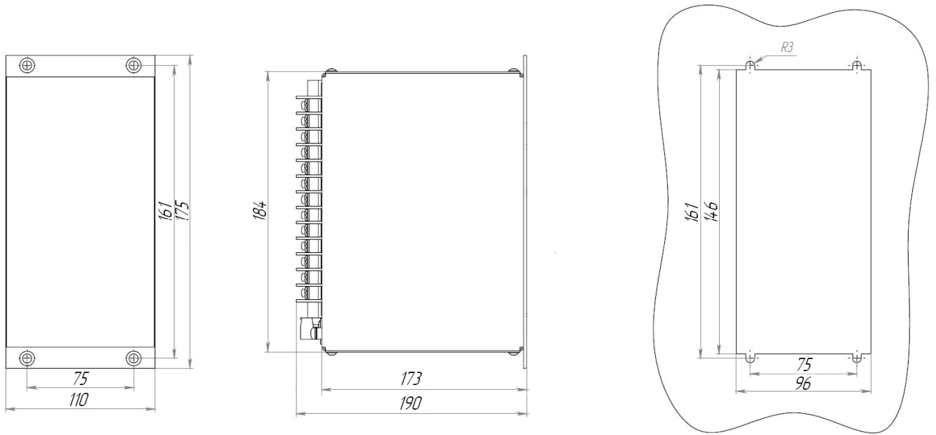
Габаритные и установочные размеры LX 120.6k.
