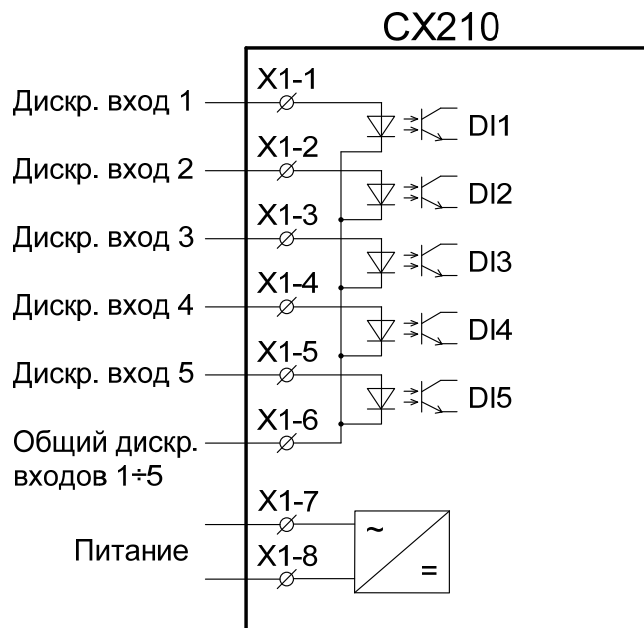
Рис. 3. Схема подключения.
