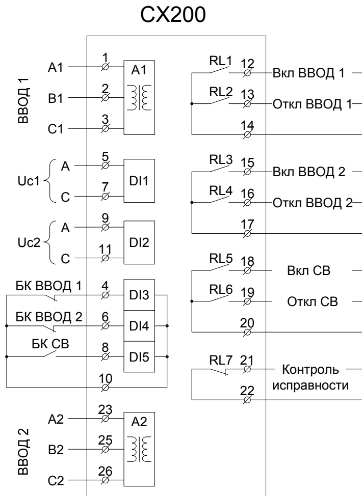
Схема подключения устройства СХ200.
